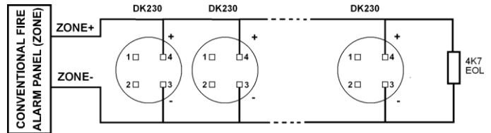
Şekil 1 – Kablolama Bağlantısı
